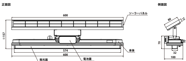
外形寸法
