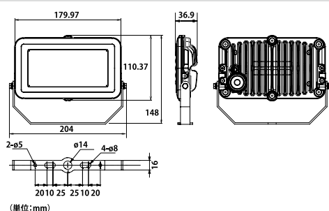
外形寸法
