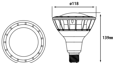
外形寸法
