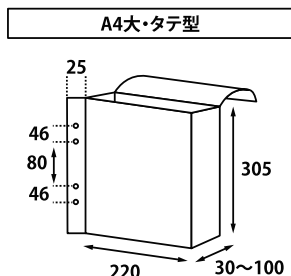
(単位:mm)
